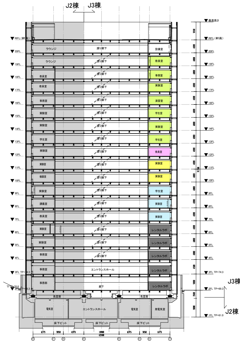
Y4-Y5通り間断面図
