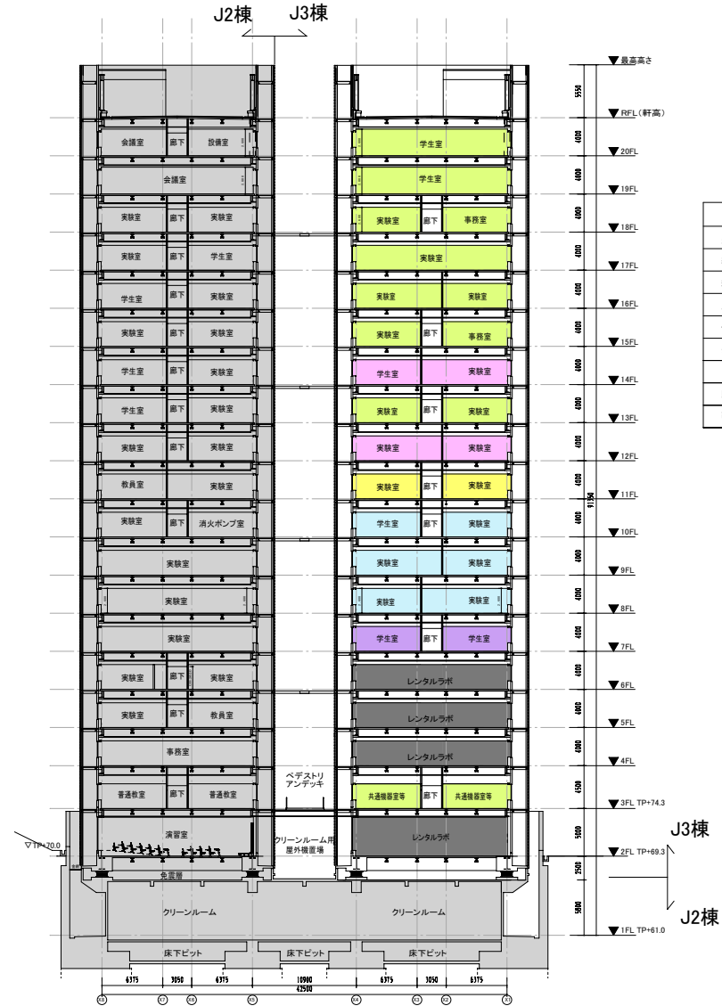
Y2-Y3通り間断面図
